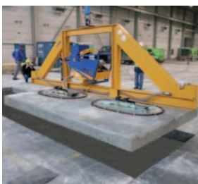
Vacuüm traverse voor buizen VT
