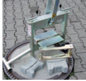
Steenknipper adapter om bochten te knippen RSA
