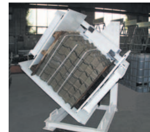
Hydraulische palletdraaitafel WT-P
