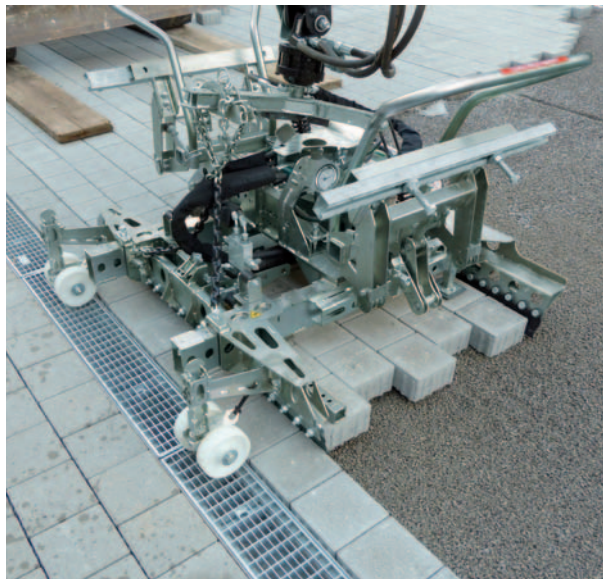
HVZ-ECO Hydraulische bestratingstang
